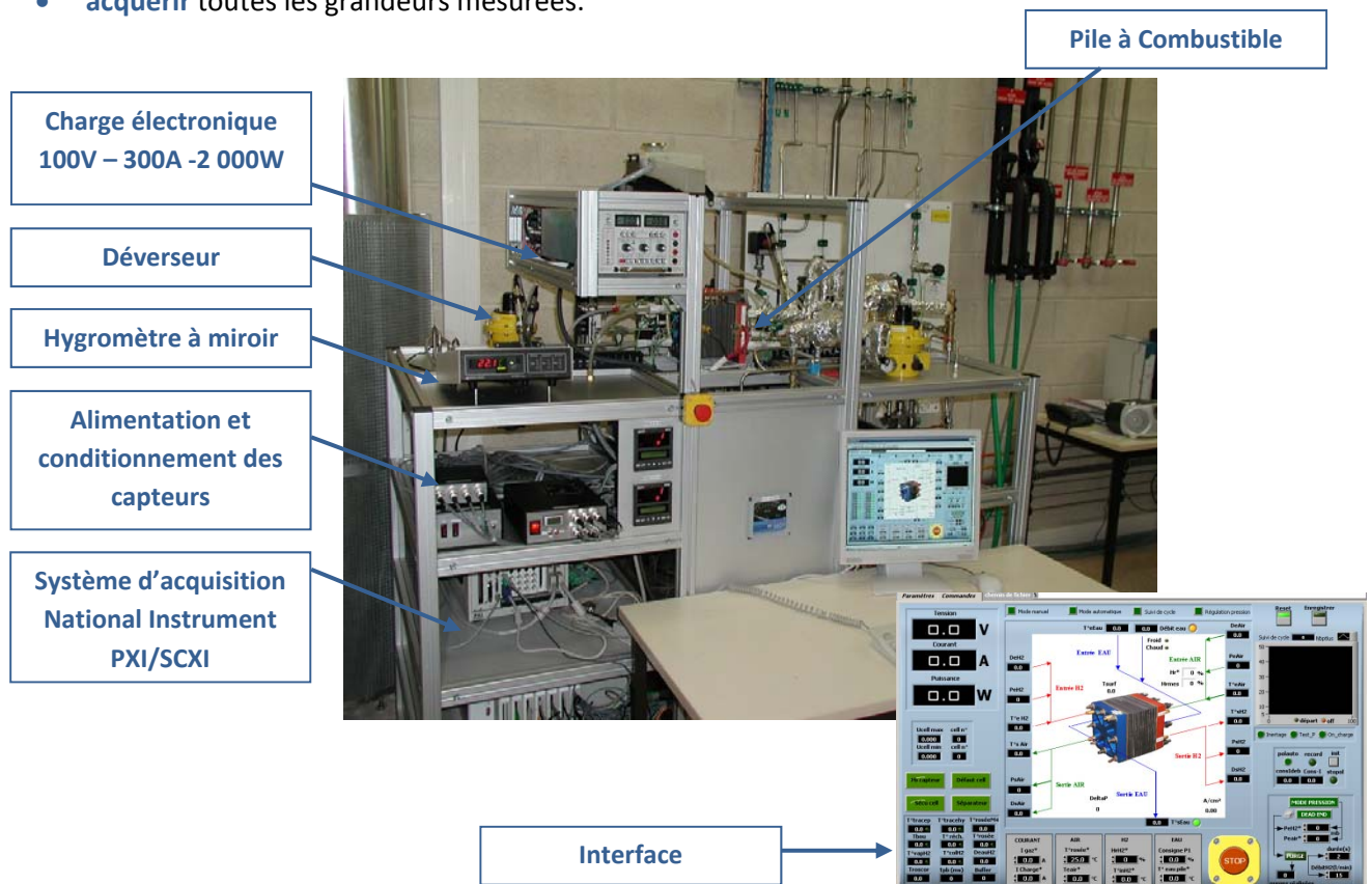
Figure 1 : Banc d'essais expérimental Pile à Combustible de type PEM \leq 1 kW.
